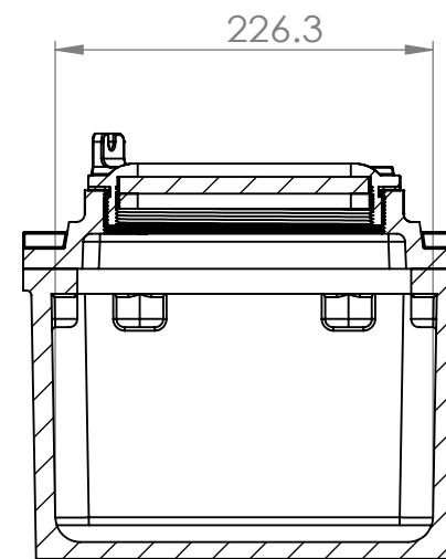
剖面圖 B-B
