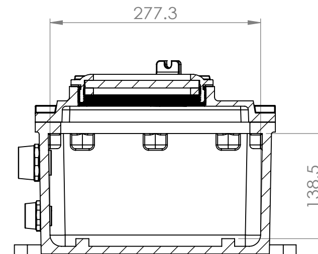
剖面圖 A-A
